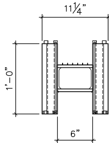
6" GBLOX (END VIEW)
