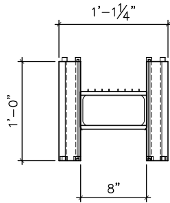
8" GBLOX (END VIEW)
