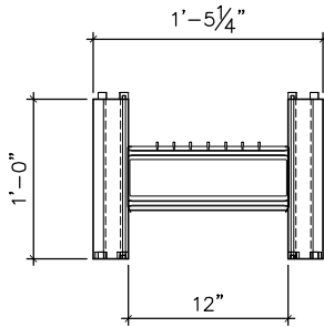
12" GBLOX (END VIEW)
